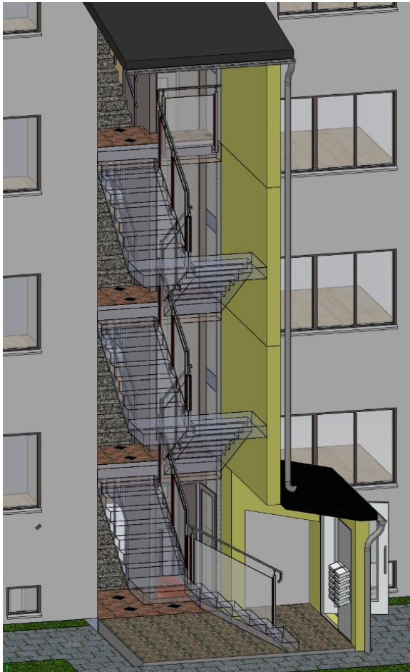
Sicht in das Treppenhaus mit Lage Aufzug
